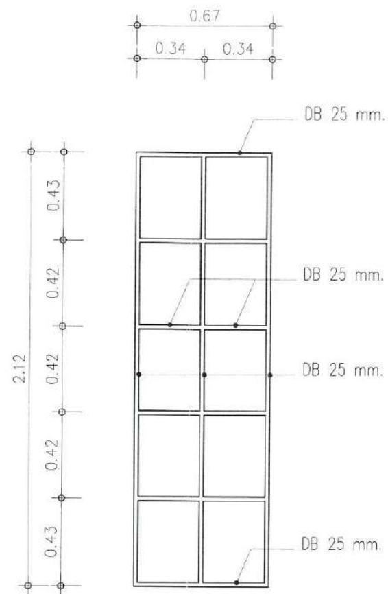
แปลนตะแกรงเหล็ก มาตราส่วน 1 : 25
