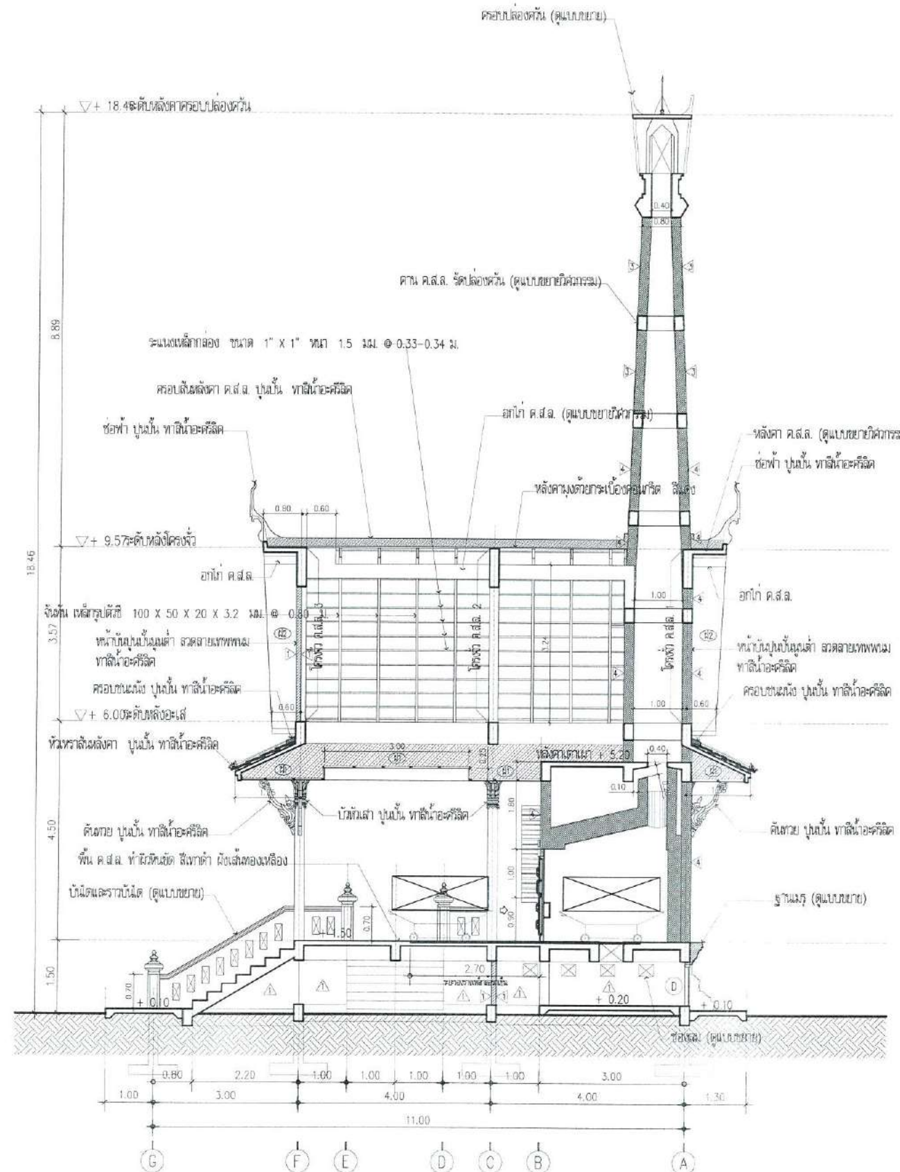
แบบแสดง ขนาดส่วน รูปตัด B. 1:100
