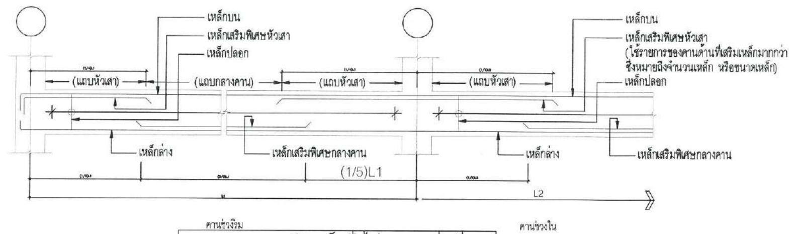
แบบแสดงการเสริมเหล็กทั่วไปของคานต่อเนื่อง
