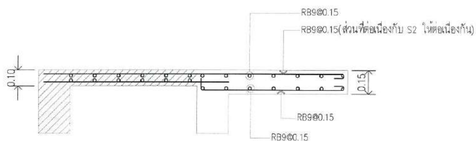
แบบแสดง แบบขยายพื้น คสล. S3
