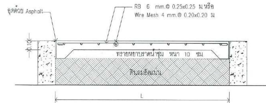
แบบแสดง ขยายพื้น GS SCALE 1:25
