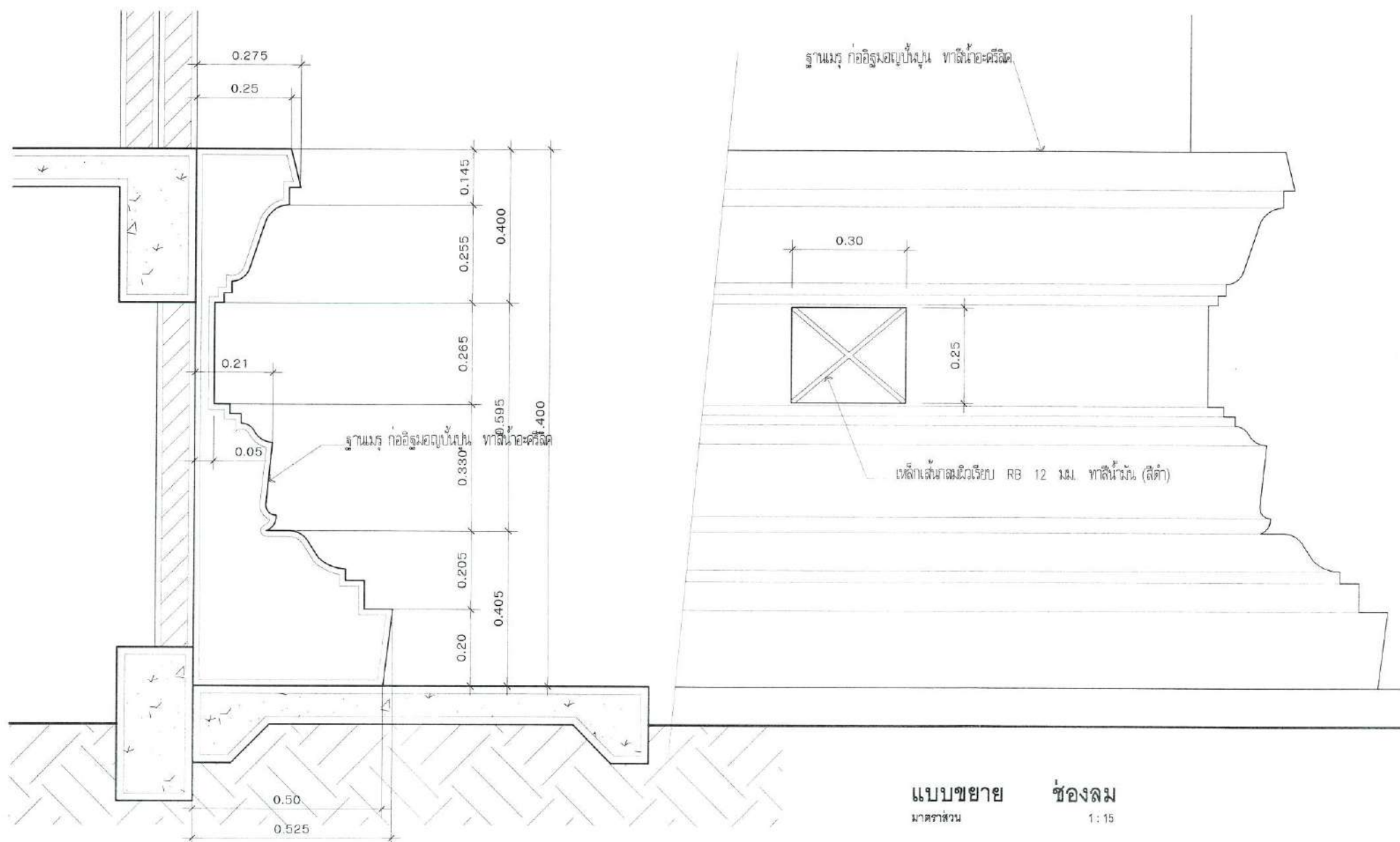
แบบขยาย ฐานเมรุ มาตราส่วน 1:15
