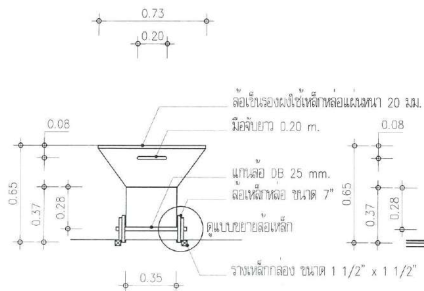
รูปด้านหน้ารถเข็น มาตราส่วน 1 : 25
