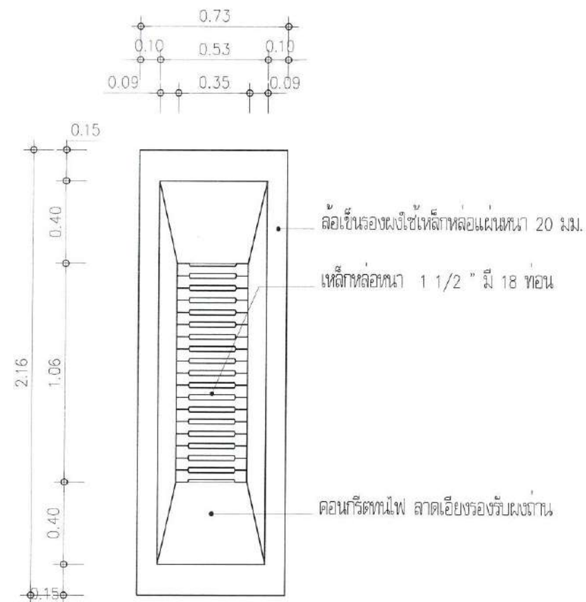
แปลนลวดเส้น มาตราส่วน 1 : 25
