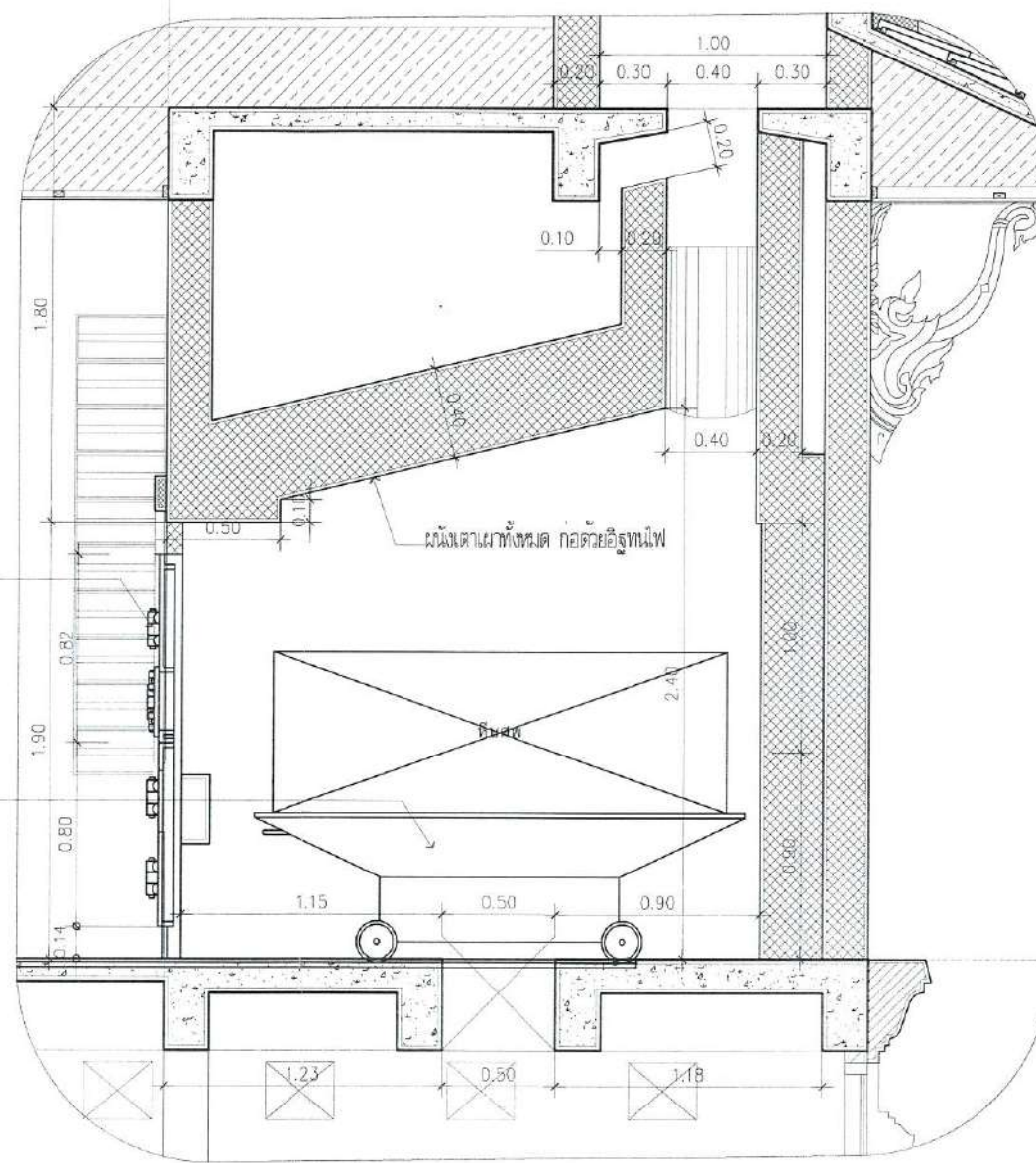
แบบแสดง รูปตัด 2. มาตราส่วน 1 : 30
