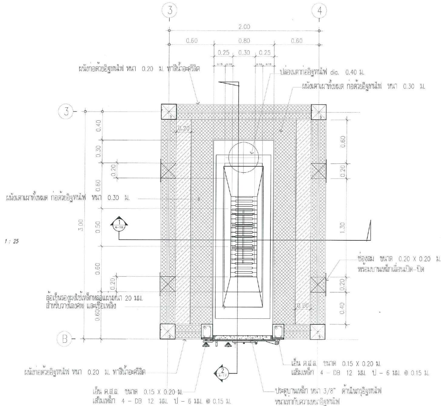
แบบแสดง แปลนเตาเผา มาตราส่วน 1:25
