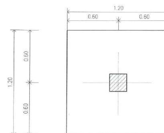
แบบขยายฐานราก F2 SCALE 1:25
