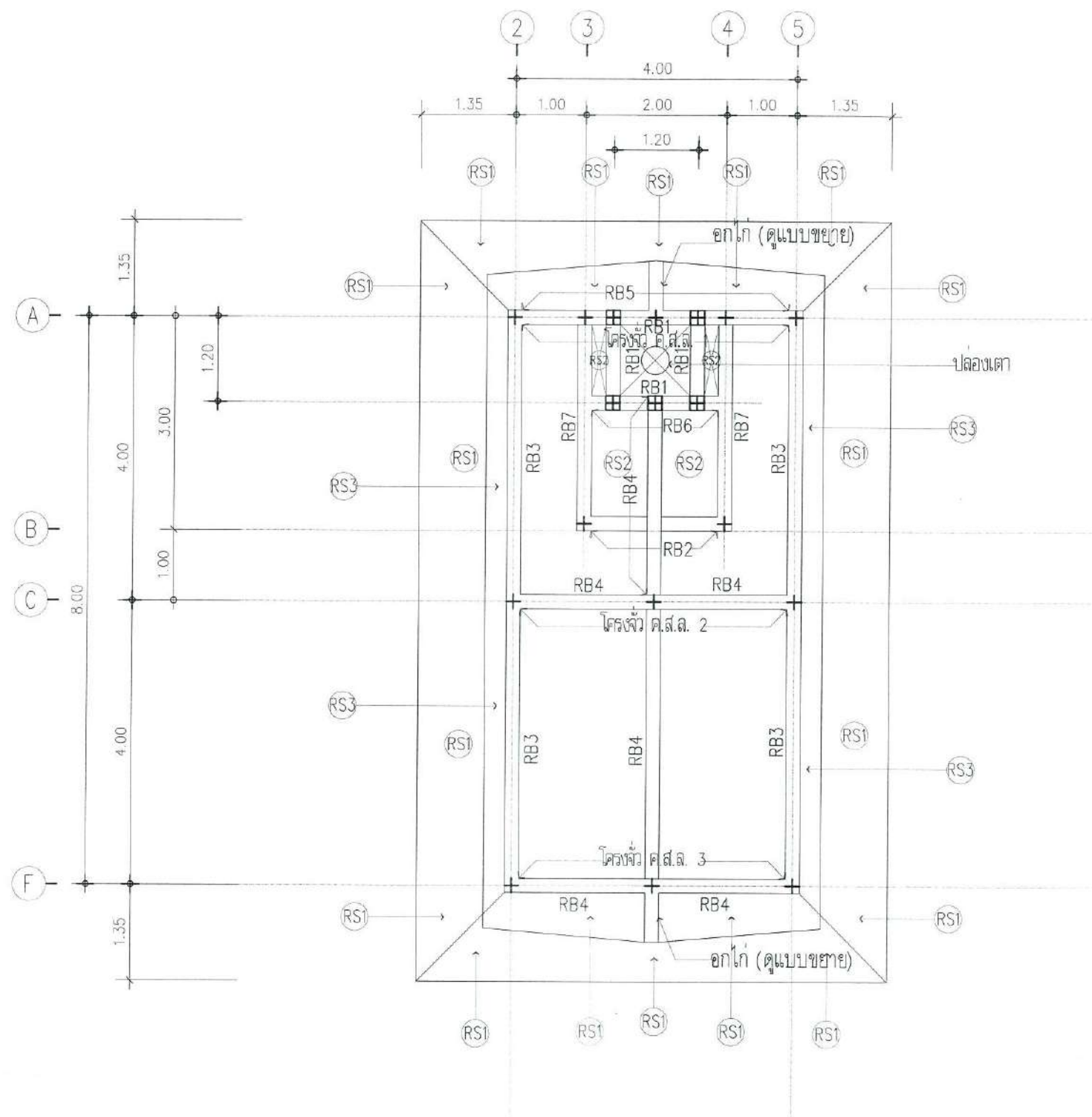
แบบแสดง ผังโครงสร้างคานชั้นหลังคา มาตราส่วน 1 : 75
