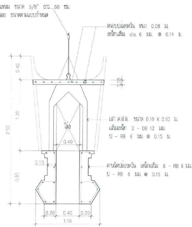
รูปตัด ก.
