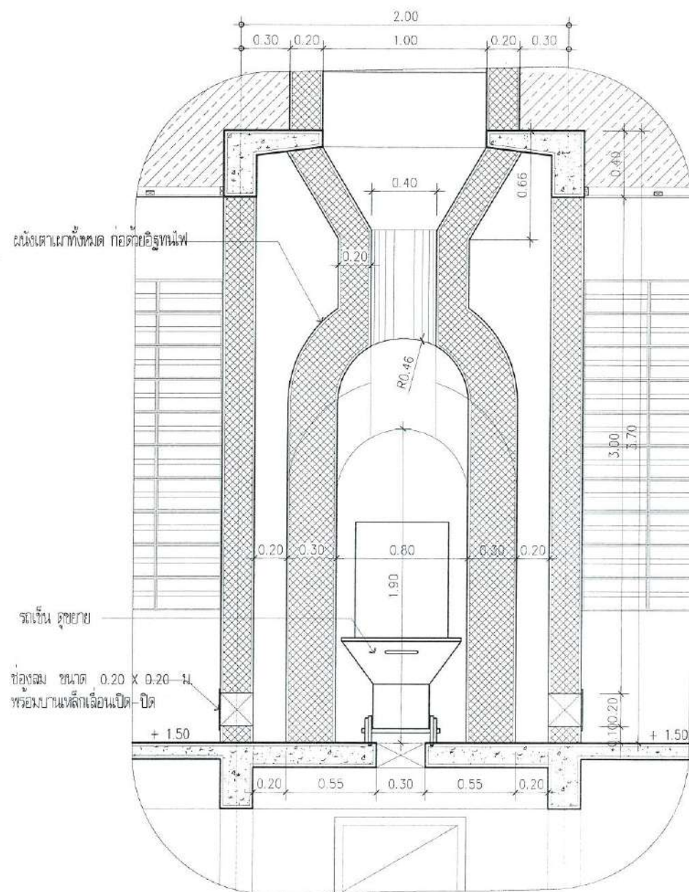
แบบแสดง รูปตัด 1. มาตราส่วน 1 : 30
