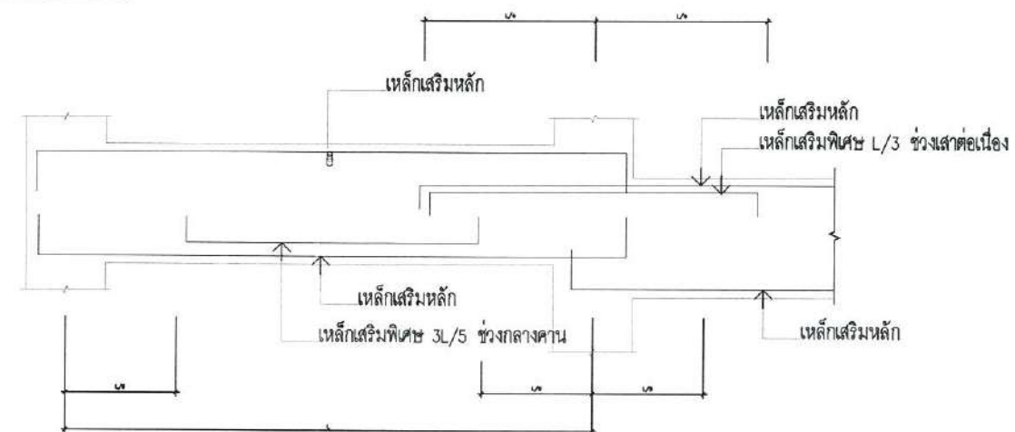
แบบแสดงเหล็กเสริมพิเศษในคานต่างระดับ
