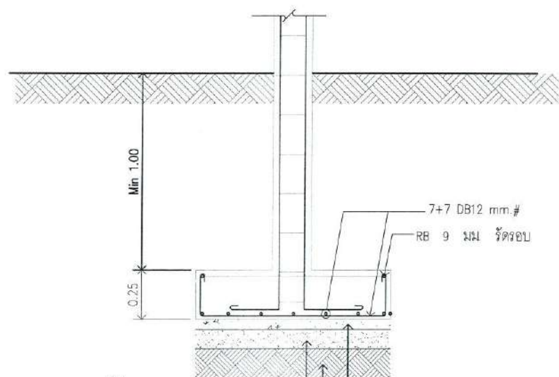
แบบขยาย รานราก F3 SCALE 1:25
