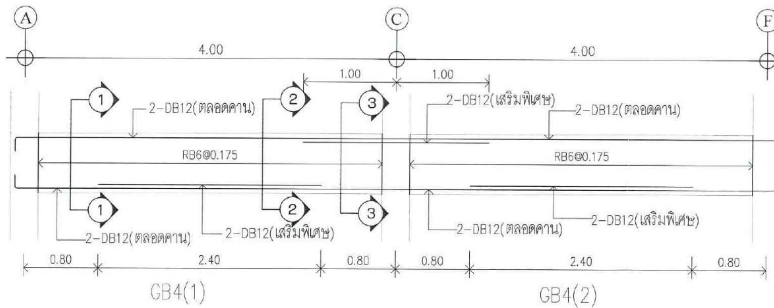
แบบขยายรูปตัดทางยาว GB4 ขนาดคาน (0.20x0.40)
