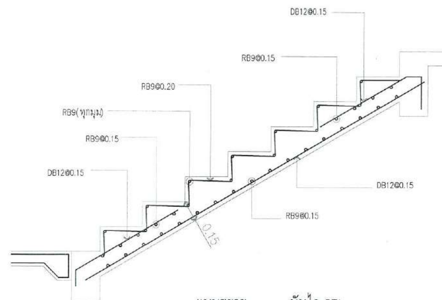
แบบขยาย บันได ST1 SCALE 1:25
