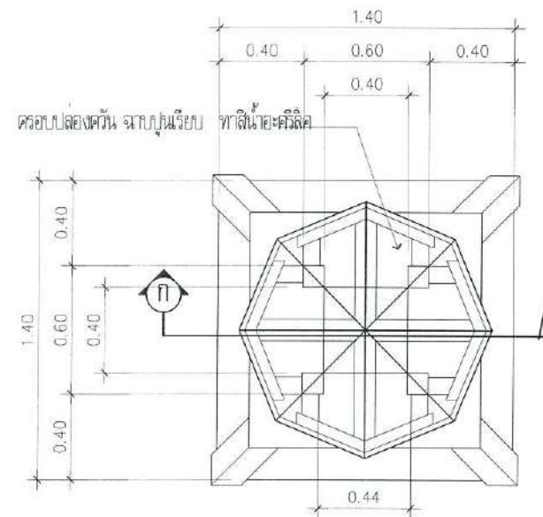
แปลนปล่องควัน
