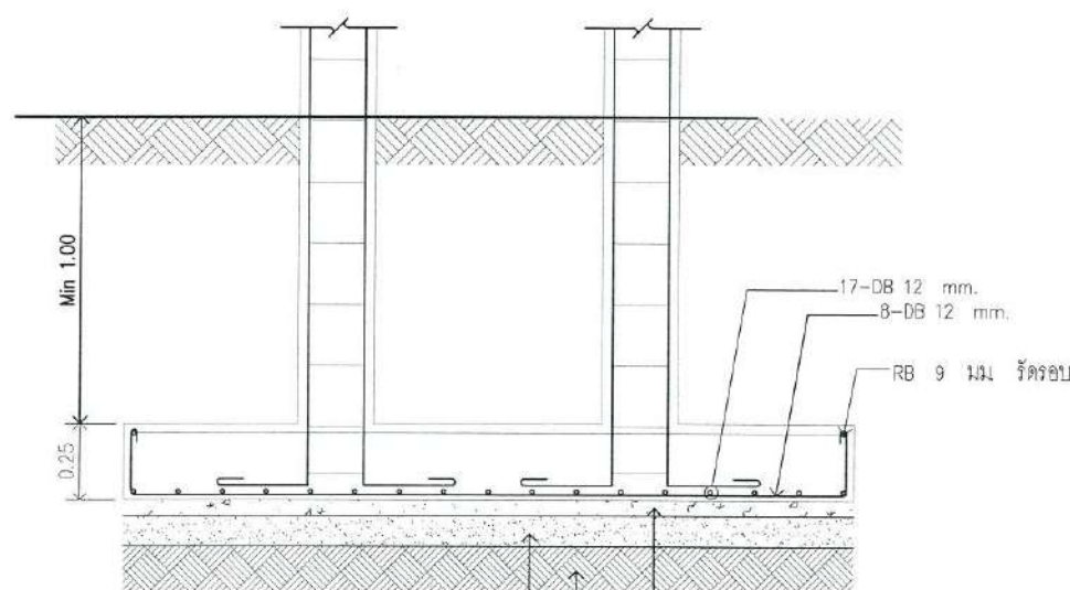
แบบขยายฐานราก F1 SCALE 1:25
