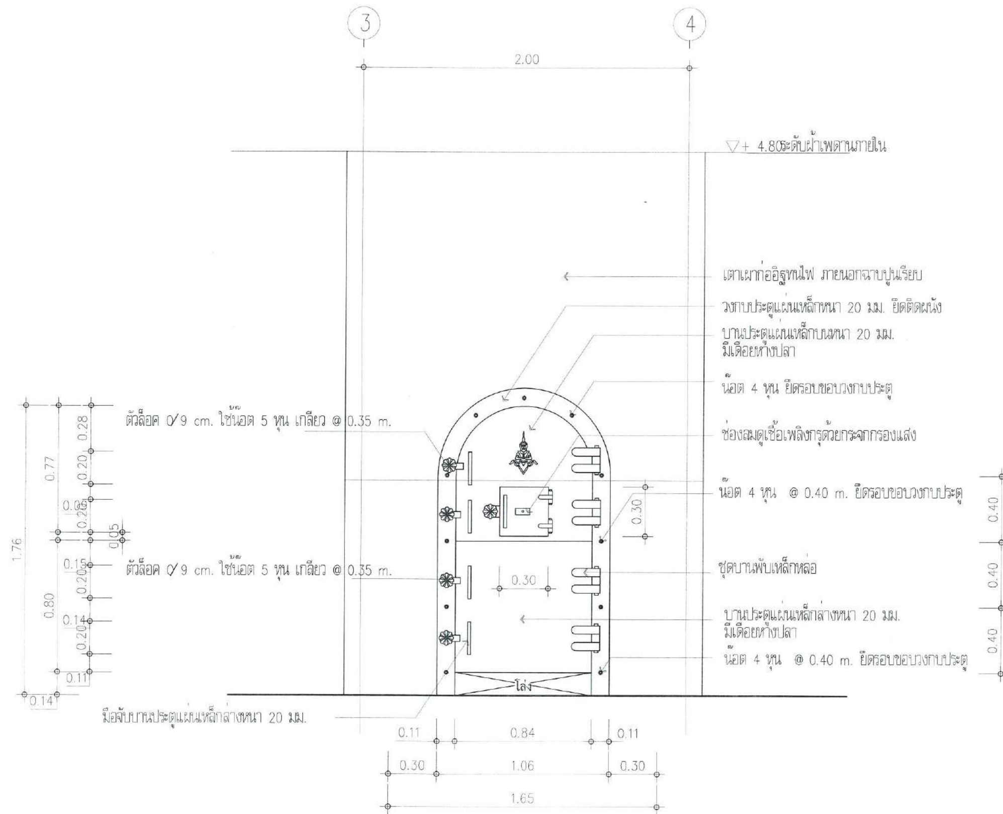
แบบแสดง รูปด้านหน้าเตาเผา มาตราส่วน 1 : 25
