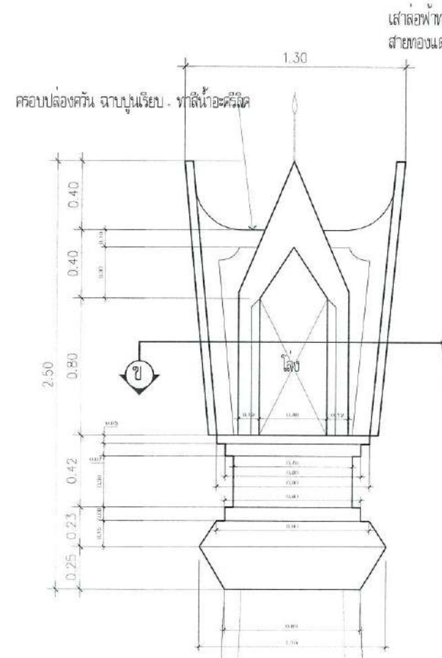
รูปตัด ข.
