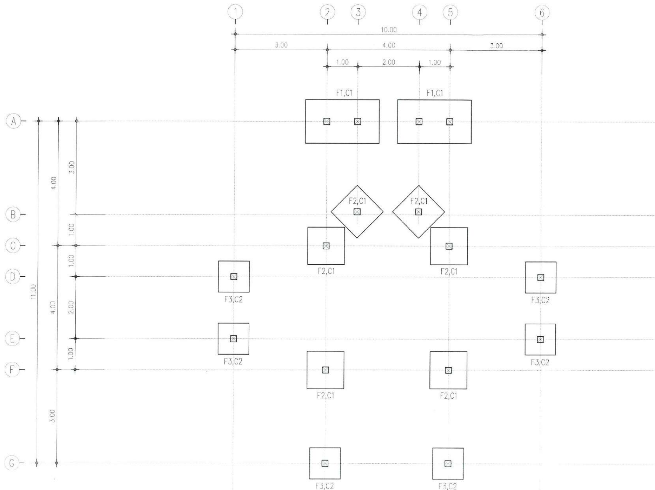
แบบแสดง มาตราส่วน ผังโครงสร้างฐานราก 1 : 75
