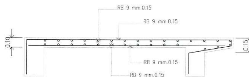
แบบขยาย SCALE พื้น RS2(ระดับ +5.20) 1:25
