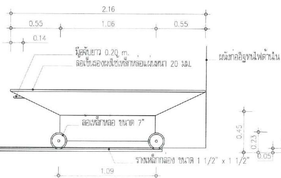
รูปด้านข้างรถเข็น มาตราส่วน 1 : 25
