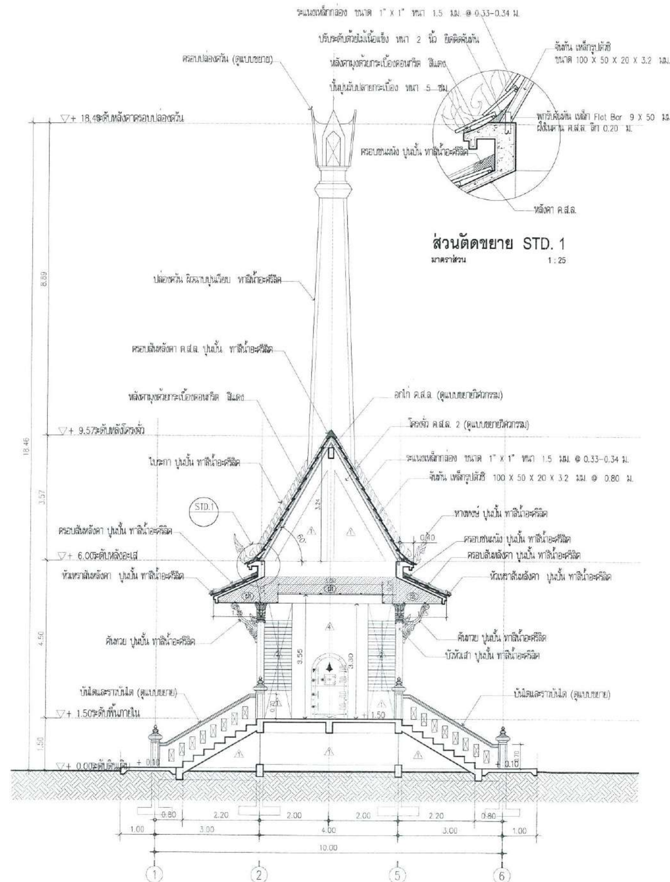
แบบแสดง รูปตัด A. มาตราส่วน 1 : 100
