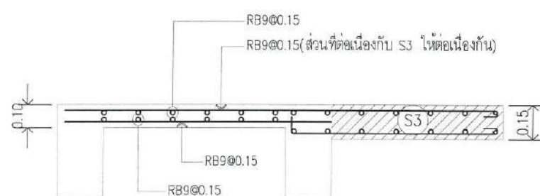
แบบแสดง แบบขยายพื้น คสล. S2
