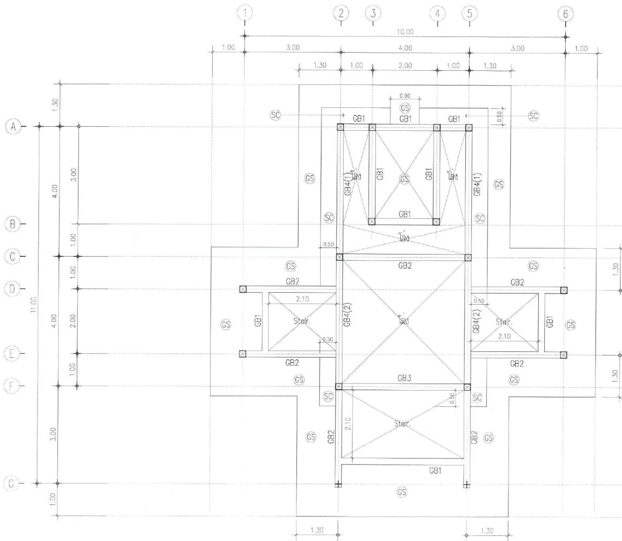
แบบแสดง มาตราส่วน ผังโครงสร้างคานคอดิน 1:75
