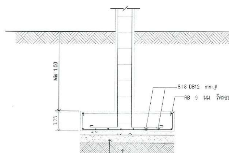
แบบขยายฐานราก F2 SCALE 1:25
