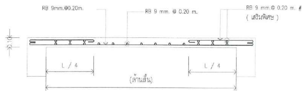
แบบแสดง แบบขยายพื้น คสล. S1
