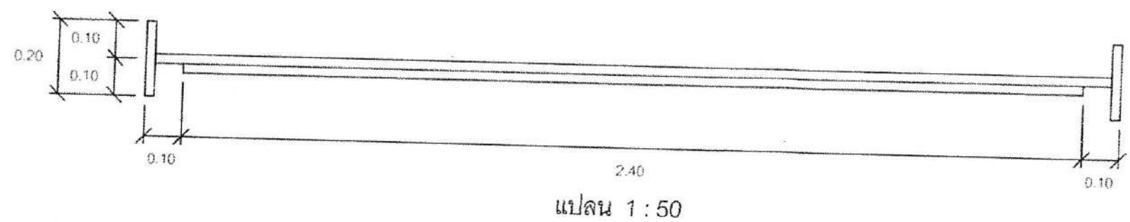
รูปด้านหน้า 1 : 50
