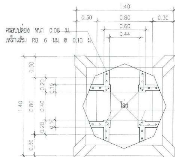
รูปตัด ข.
